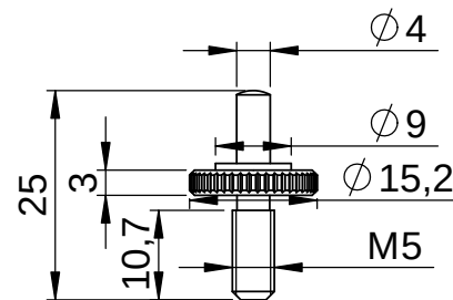
Höhenverstellschraube level adjustable screw
