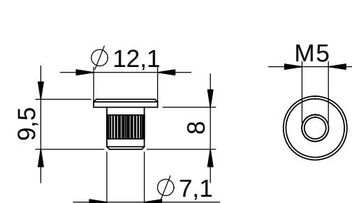
Einschlagmutter insert
